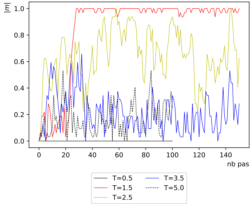
Evolution selon critère Estimation par intervalle,Condition Initiale alterné 4lignes-4lignes, Réseau taille L=8
